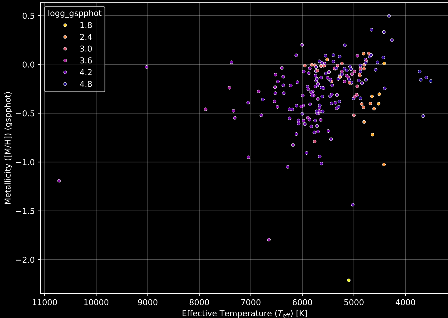
APOGEE DR17 Field: [105-30] Stellar Population Parameters (n= 195)
